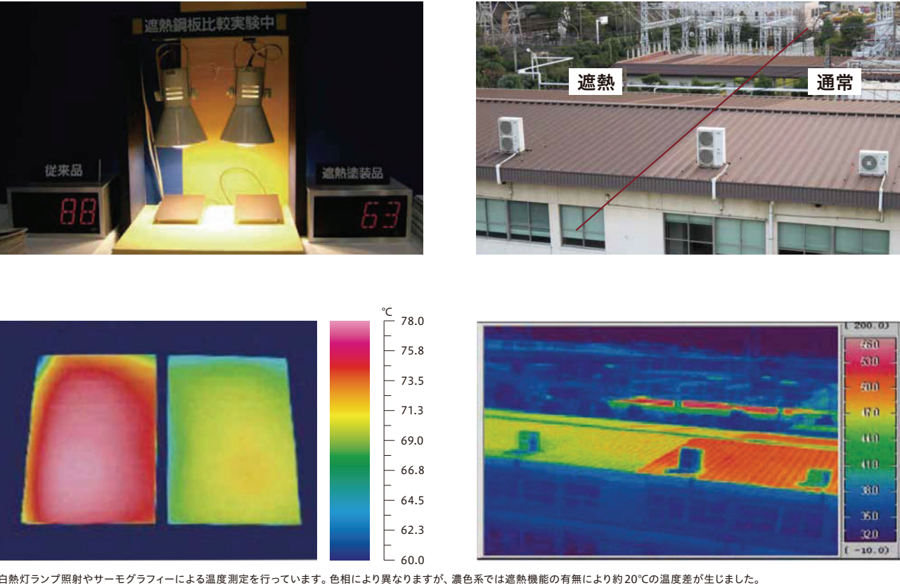
白熱灯ランプ照射やサーモグラフィーによる温度測定を行っています。色相により異なりますが、濃色系では遮熱機能の有無により約20℃の温度差が生じました。
